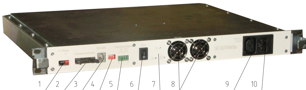
Рисунок 2.3 - Инвертор Штиль PS48-60/1000
