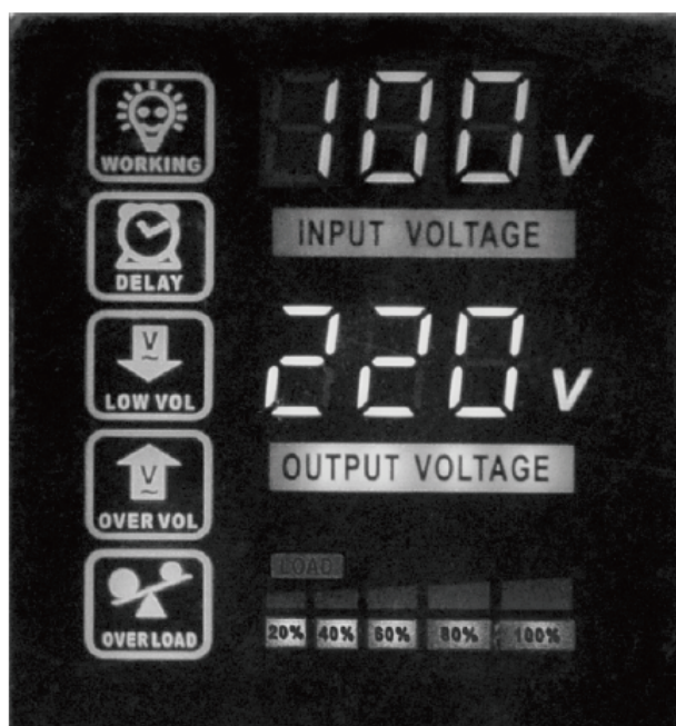
Рис. 3 Мультифункциональный цветной дисплей
