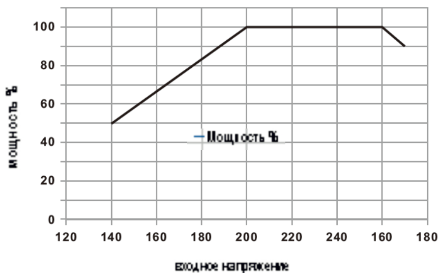
Рис. 2 График зависимости выходной мощности стабилизатора от входного напряжения.
