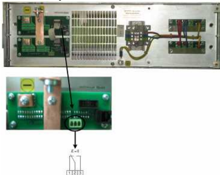
Рисунок 1.9 – Расположение сигнального разъема на ответной плате горячего включения, для инверторов Штиль PS 60/1500(HS) и Штиль PS 60/1500(HS-STS)
